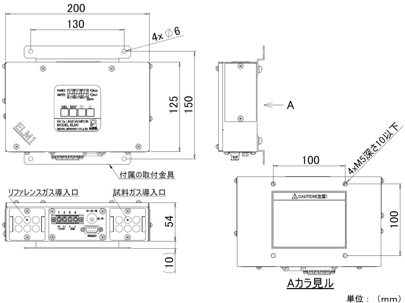
図-4 取付け穴ピッチ図
