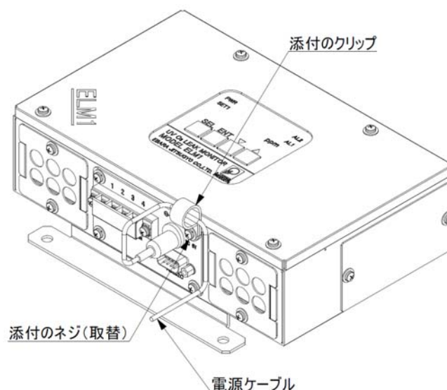
図-5 電源ケーブルの抜け止め対策
